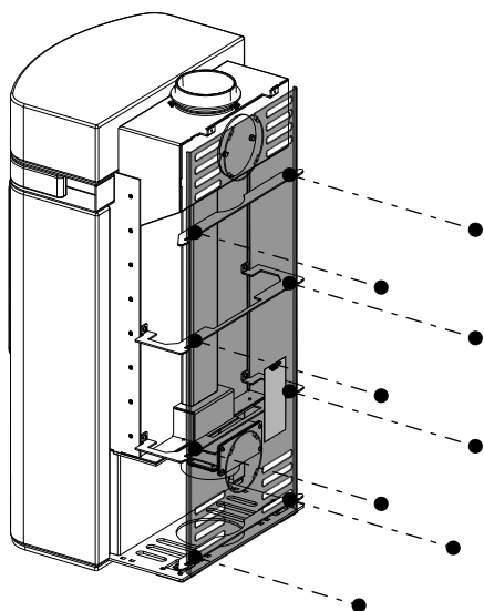
Fig. 14: Rimozione della parete posteriore
