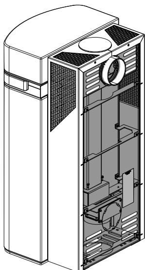
Fig. 13: Rimontaggio della parete posteriore
