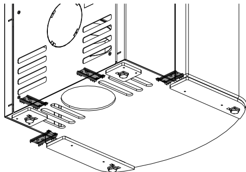
Fig. 6: Rimozione dei fermi di trasporto (vista dal basso)
