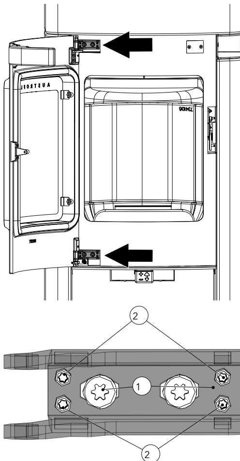
Fig. 35: Viti di registro dello sportello
