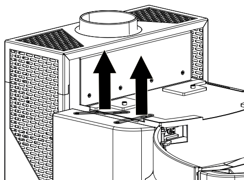
Fig. 51: Rimozione dei supporti
