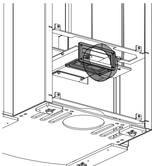
Fig. 19: Collegamento dell'aria posteriore
