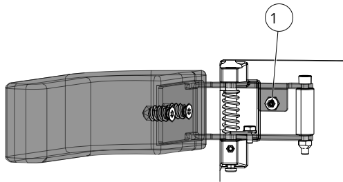
Fig. 31: Regolazione della maniglia
