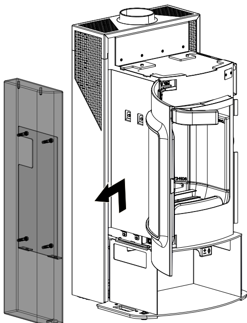
Fig. 52: Rimozione del rivestimento laterale sinistro
