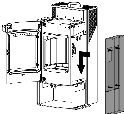
Fig. 25: Agganciamento del rivestimento laterale destro
