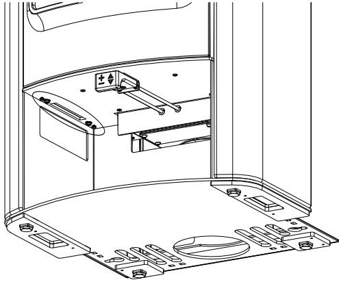
Fig. 36: Viti di regolazione del rivestimento laterale
