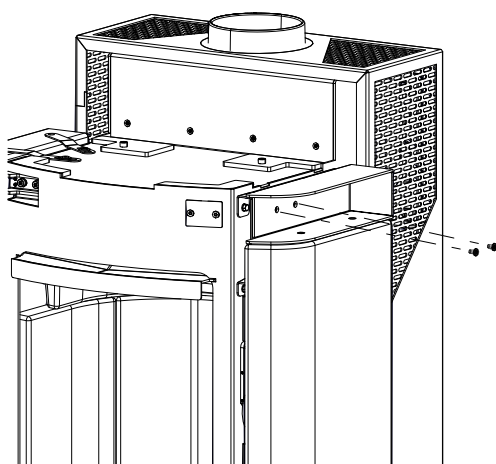
Fig. 27: Fissaggio del rivestimento laterale destro
