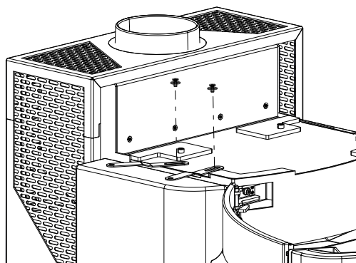
Fig. 24: Avvitamento delle viti del supporto
