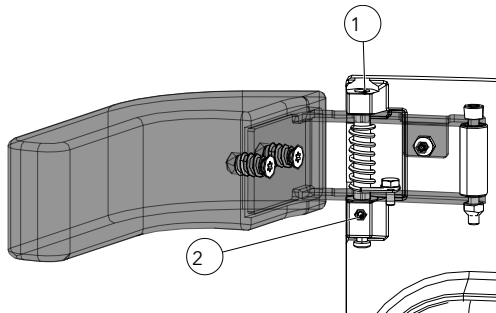
Fig. 33: Impostazione della forza di chiusura della maniglia
