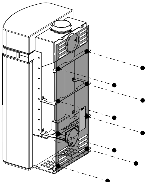
Fig. 8: Rimozione della parete posteriore
