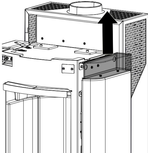
Fig. 48: Sollevamento della scatola con la maniglie
