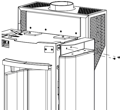
Fig. 47: Rimozione delle viti
