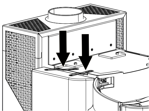
Fig. 23: Fissaggio del supporto
