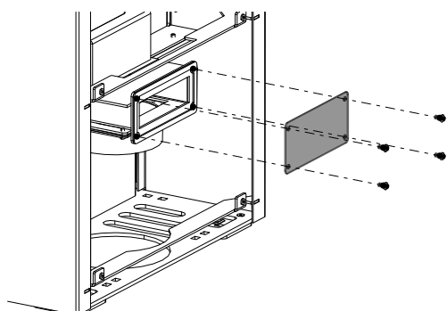
Fig. 16: Smontaggio del coperchio posteriore
