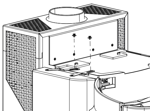
Fig. 50: Svitamento del supporto
