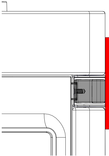
Fig. 32: Regolazione della maniglia a filo con il rivestimento laterale
