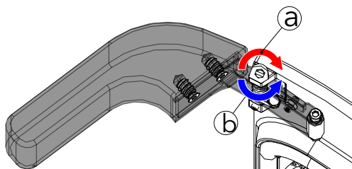
Fig. 34: Chiusura della maniglia in modo più leggero / forte
