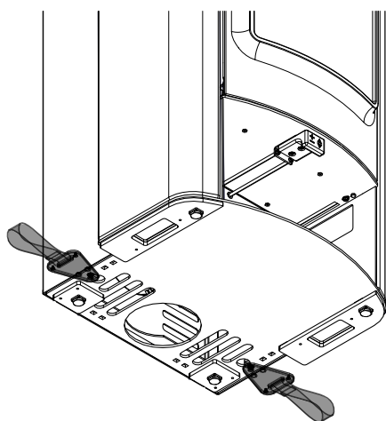
Fig. 7: Mezzo di trasporto
