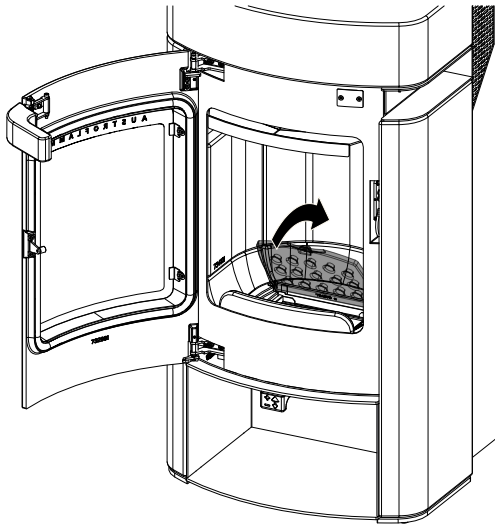
Fig. 40: Sollevamento della griglia
