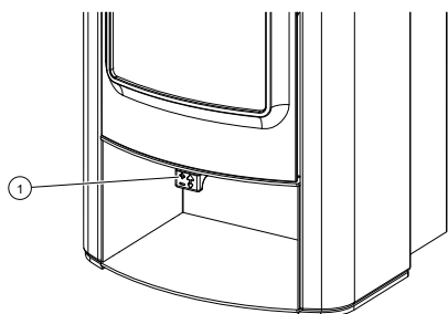
Fig. 37: Regolatore dell'aria primaria/secondaria
