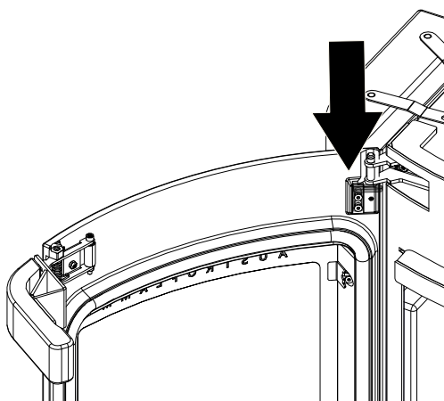
Fig. 53: Chiusura dello sportello
