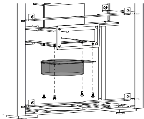
Fig. 17: Smontaggio della connessione dell'aria
