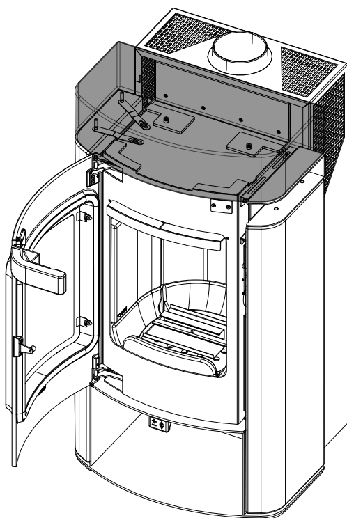
Fig. 45: Rimozione del coperchio
