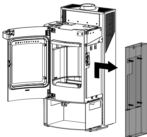
Fig. 49: Rimozione del rivestimento laterale destro
