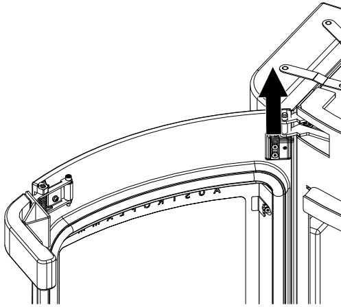
Fig. 46: Bloccaggio della la porta
