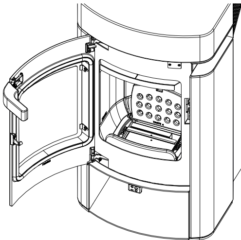
Fig. 42: Chiusura del coperchio
