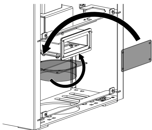
Fig. 18: Sostituzione della flangia e del coperchio
