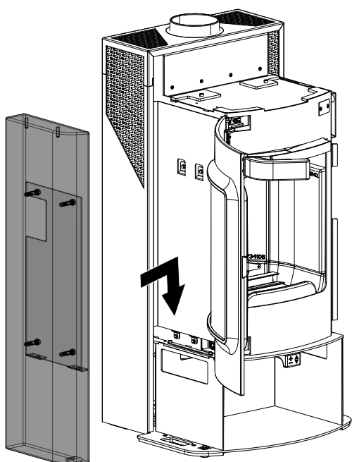
Fig. 22: Agganciamento del rivestimento laterale sinistro
