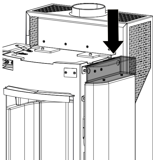
Fig. 26: Inserimento della scatola con la maniglia
